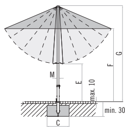
Loser Deckbelag max. 10 cm, Betondicke min. 30 cm (Frosttiefe beachten), Wasserabfluss.
